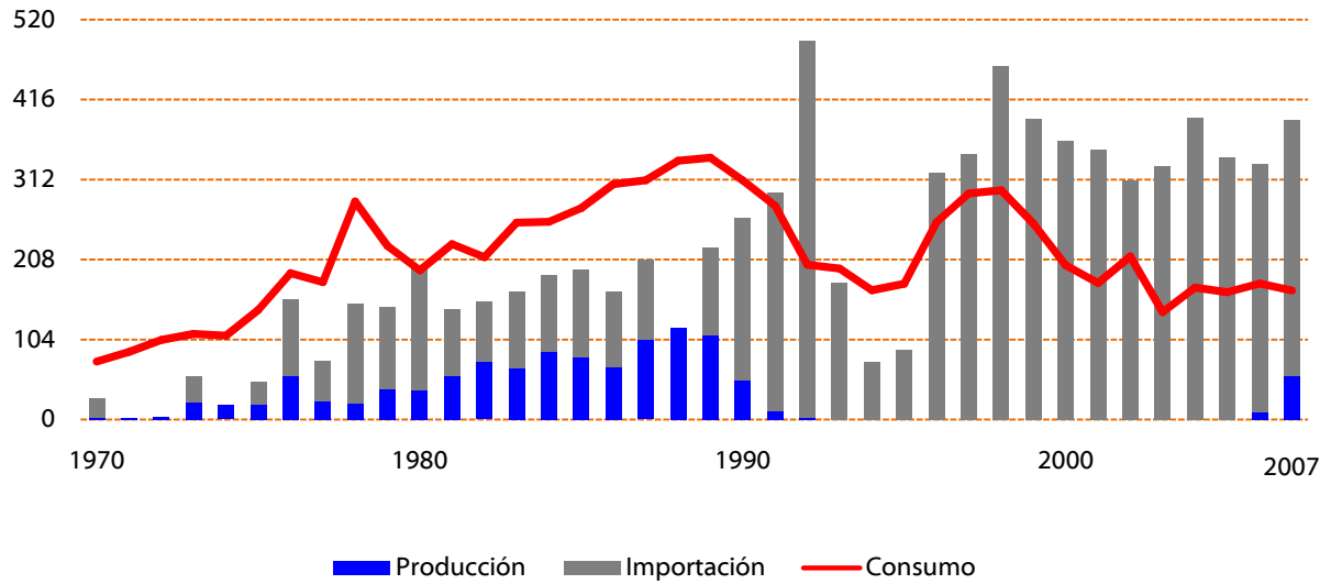
Gráfico 41. Producción, importación y consumo de Turbocombustible. Período 1970 - 2007 - Miles de toneladas -
